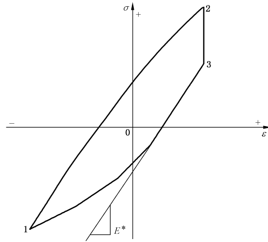
图 D.1 应变保持 \sigma - \epsilon 迟滞回线
